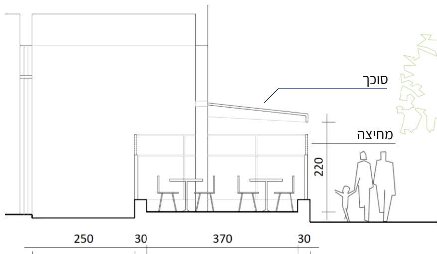
מחיצה טלסקופית על גבי במה
