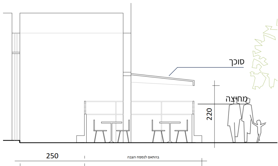
מחיצה טלסקופית על גבי מדרכה
